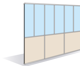
Vitré traverses verticales sur allège pleine
